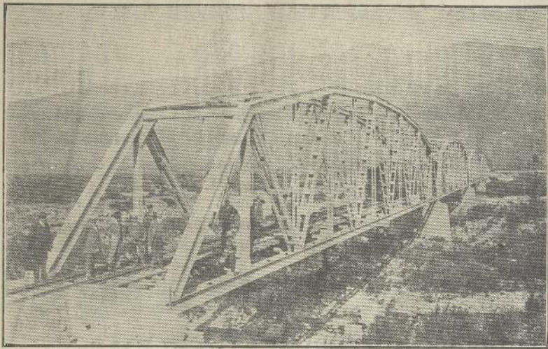
Puente sobre el río Petorca.—Cuatro tramos de 60 metros y uno de 30
