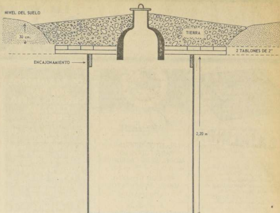
Esquema de pozo cubierto.
