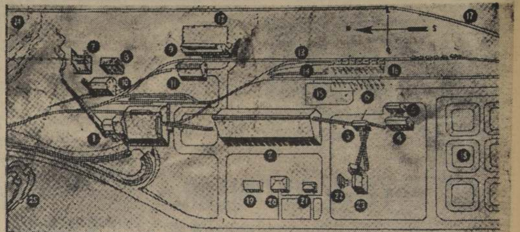
PLANO DE LA FUNDICION NACIONAL DE PAIPOSE. — Los números indican: 1, la fundición; 2, tolvas de mezclas; 3, casas de distribución; 4, planta trituradora; 5, casas de distribución; 6, receptor de minerales; 7, subestación de energía eléctrica; 8, torres de enfriamiento; 9, bodega; 10, la planta de energía eléctrica; 11, la casa de máquinas; 12, patio de almacenaje y materiales; 13, empalmes de vías ferreas; 14, stock de carbón; 15, almacenaje de concentrados y secador; 16, stock de carbón; 17, Ferrocarril Norte 18; patios para minerales; 19, garage; 20, oficina; 21, laboratorio; 22, casa de distribución; 23, planta de muestras; y 24, línea eléctrica a Copiapó.
