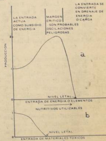
Fig. N° 3 Efecto de niveles crecientes de contaminantes biodegradables (A) y no degradables (B) sobre el ecosistema.
