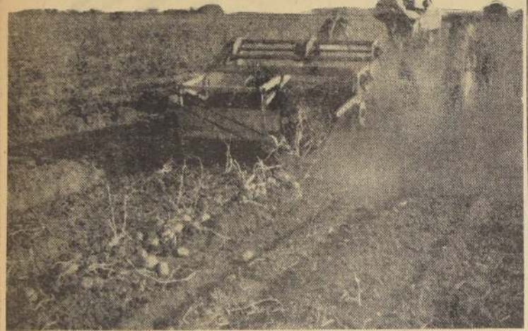
El hilerador, de montaje en la parte posterior de esta arrancadora para dos surcos, coloca las papas en una sola hilera.
