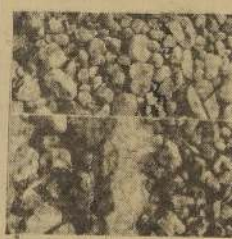
Fotografía de un agregado grueso, perfectamente graduado, antes y después de haberlo clasificado en tres tamaños. Se puede observar que los agregados pequeños ocupan todos los huecos de los más grandes.
