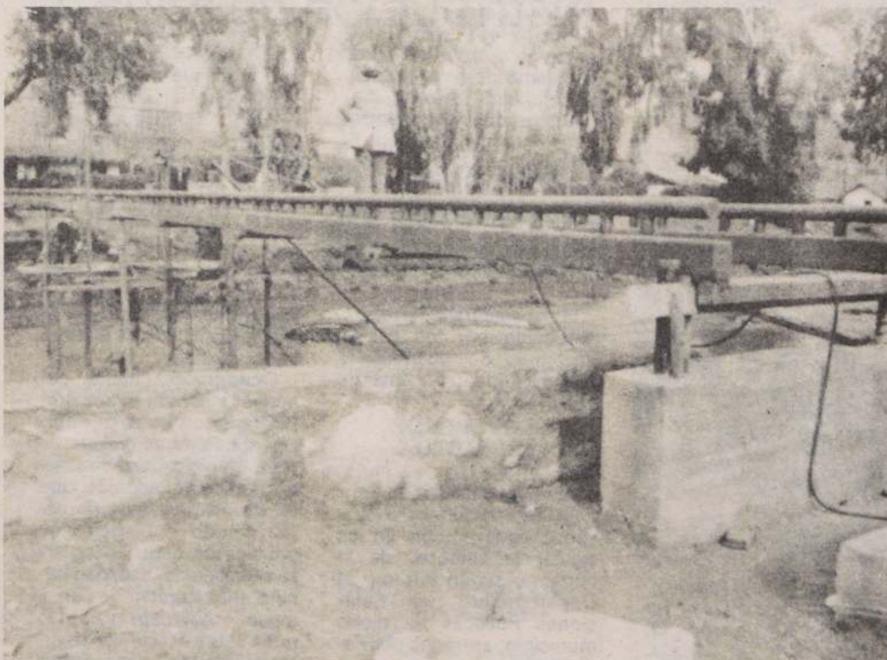
LEVANTAN PUENTE PARA PEATONES destruido por aguas del estero de Reñaca y que dejó aisladas a dos poblaciones de la parte alta. En la fotografía, parte de la estructura.
