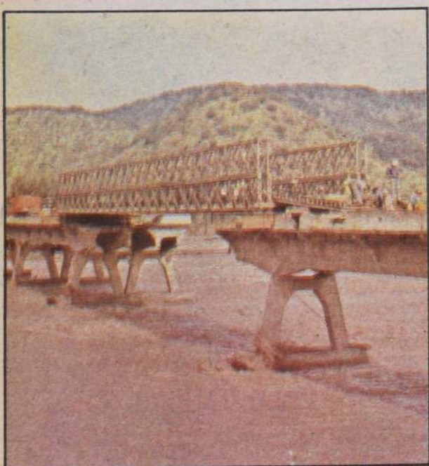
PUENTE DE EMERGENCIA.— Vehículos de hasta 30 toneladas, incluyendo buses, podrán cruzar el viaducto metálico, del tipo Bailey, sobre el río Tinguiririca, junto a San Fernando, que fue habilitado por efectivos de la Escuela de Ingenieros Militares de Tejas Verdes y personal de la Dirección de Vialidad. En la instalación se usaron las bases del puente dañado, para sustentar la estructura de 30 metros de largo.
