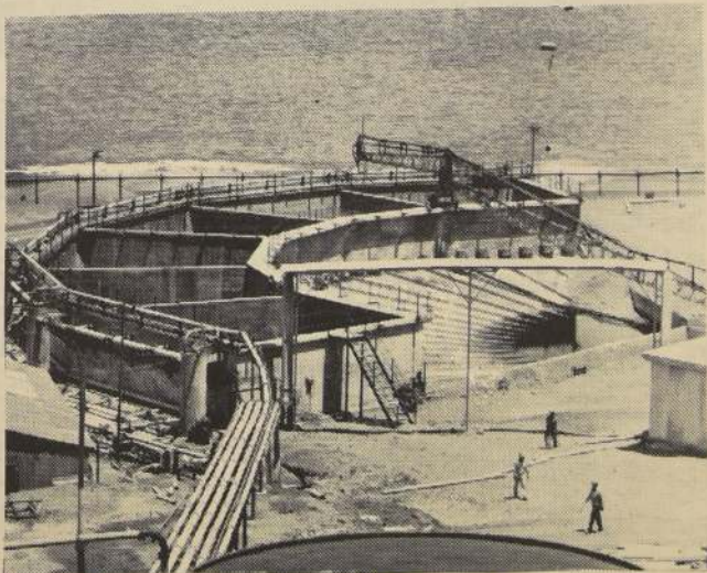
Estanques de lixiviación por percolación de la Planta "José Antonio Moreno" de ENAMI en Taltal. Este plantel, construido y puesto en marcha por el actual gobierno, fue recientemente ampliado de 3.900 toneladas mensuales de mi- nerales a 18.000 toneladas mensuales.
