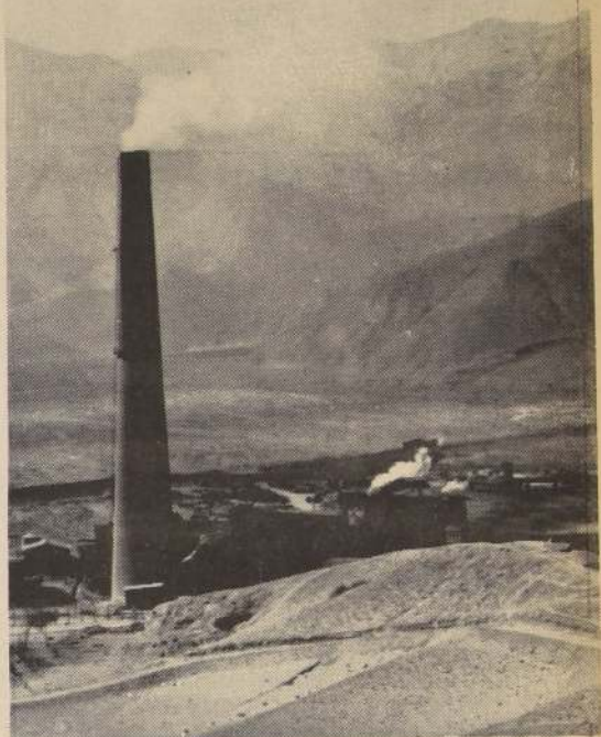
Lien mil toneladas de cobre blister producirán, hacia 1973, las Fundiciones de Paipote y Ventanas de ENAMI. En el grabado, aspecto parcial de las in- stalaciones de la primera de las usinas citadas en la que se efectúan obras de ampliación para elevar la capacidad de 24.000 a 36.000 toneladas anua- les de blister.
