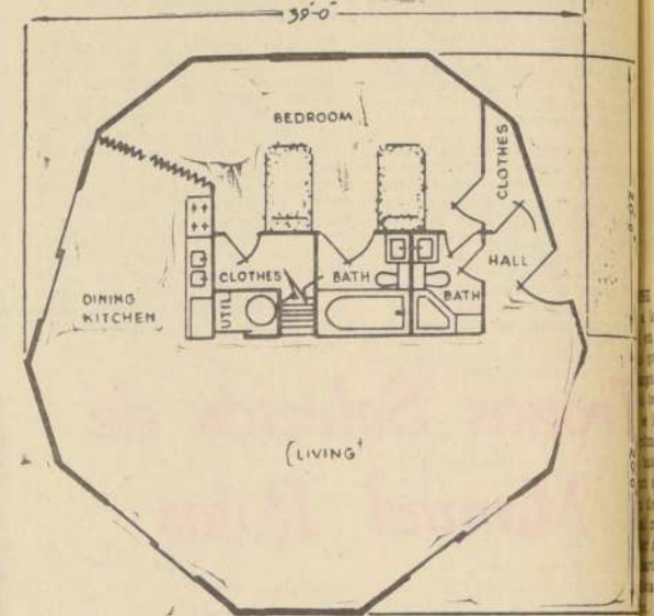
El plano del hogar de Fuller ilustra lo espaciosa que puede resultar una casa pequeña cuando no está dividida por tabiques. Sólo el dormitorio, el núcleo central, que contiene las cañerías, la instalación de calefacción y closets, están limitados por paredes interiores. La sala asciende hacia el techo de la cúpula, pero sobre todo el resto del espacio del primer piso hay una galería que contiene una biblioteca, un área de utilidad general, y, a veces, hasta alojamiento para un huésped.
