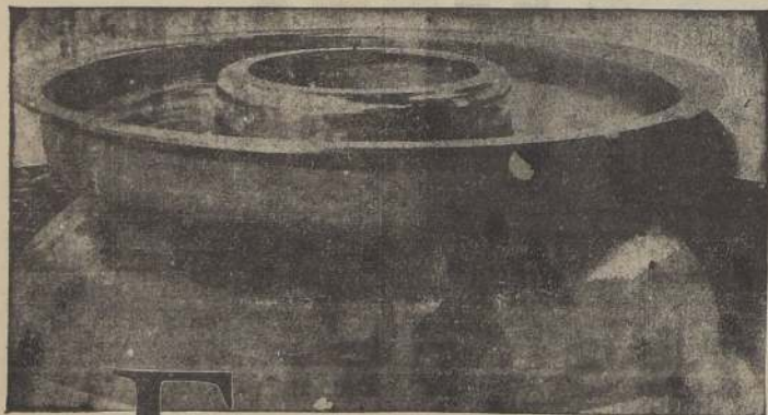
Paño para la preparación de una sola plancha de 19 mm. por la Lukens Steel Company (E. U.) para la E. I. du Pont de Nemours Co. (E. U.) Peso, 1360 kilos; diámetro, 3.25 metros.
