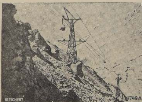
Andarivel para el transporte de minerales en la Cordillera de los Andes. Propiedad de la Compañía Minera Disputada de Las Condes
