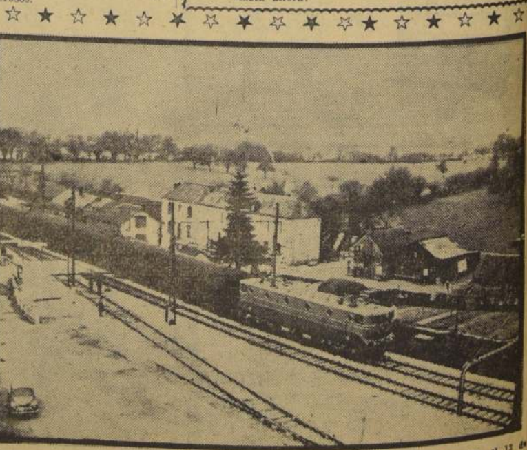
Vista del tren telegráfico, que por primera vez en la historia corrió conducido a distancia, el 13 de abril del presente año, en la línea de Mans. La máquina eléctrica es gemela de la que recientemente bató el record mundial de velocidad, y en su parte superior se distingue la antena de telemando. Aquí se ve al convoy al pasar por la estación de Sceaux-Boisse. (Foto Intercontinental).
