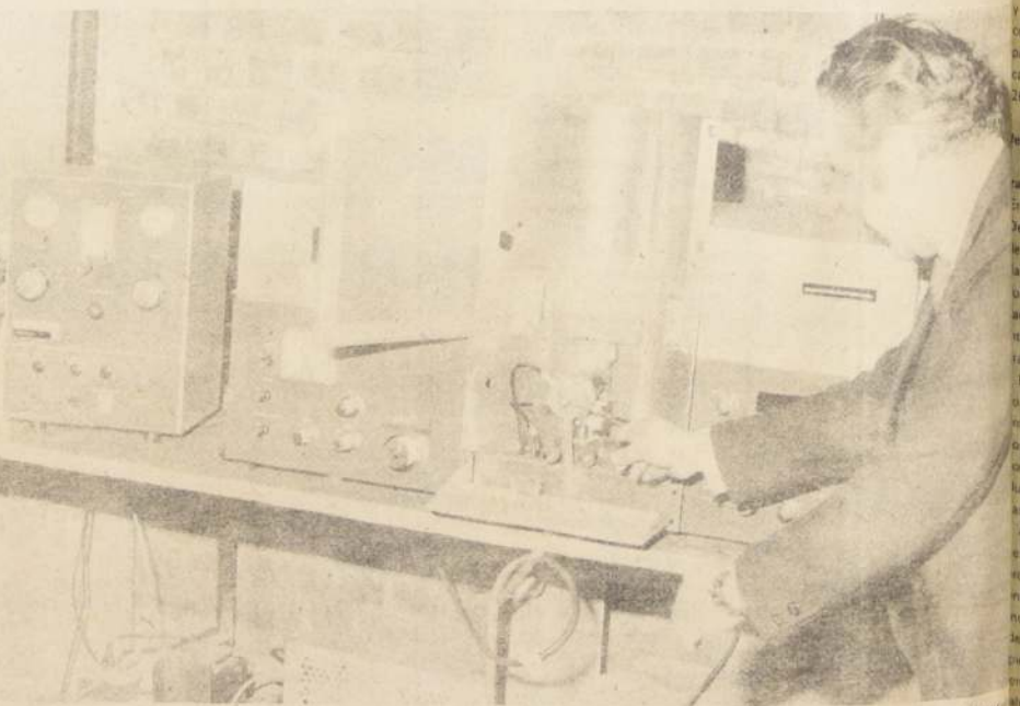
ESPECTRO-FOTOMETRO "Perkins-Elmer 403", con que cuenta la Universidad Técnica del Estado para análisis fino de cualquier elemento en solución. Donación de la empresa minera Disputada de Las Condes, a través del material analítico-instrumental en la especialidad de espectrografía.
