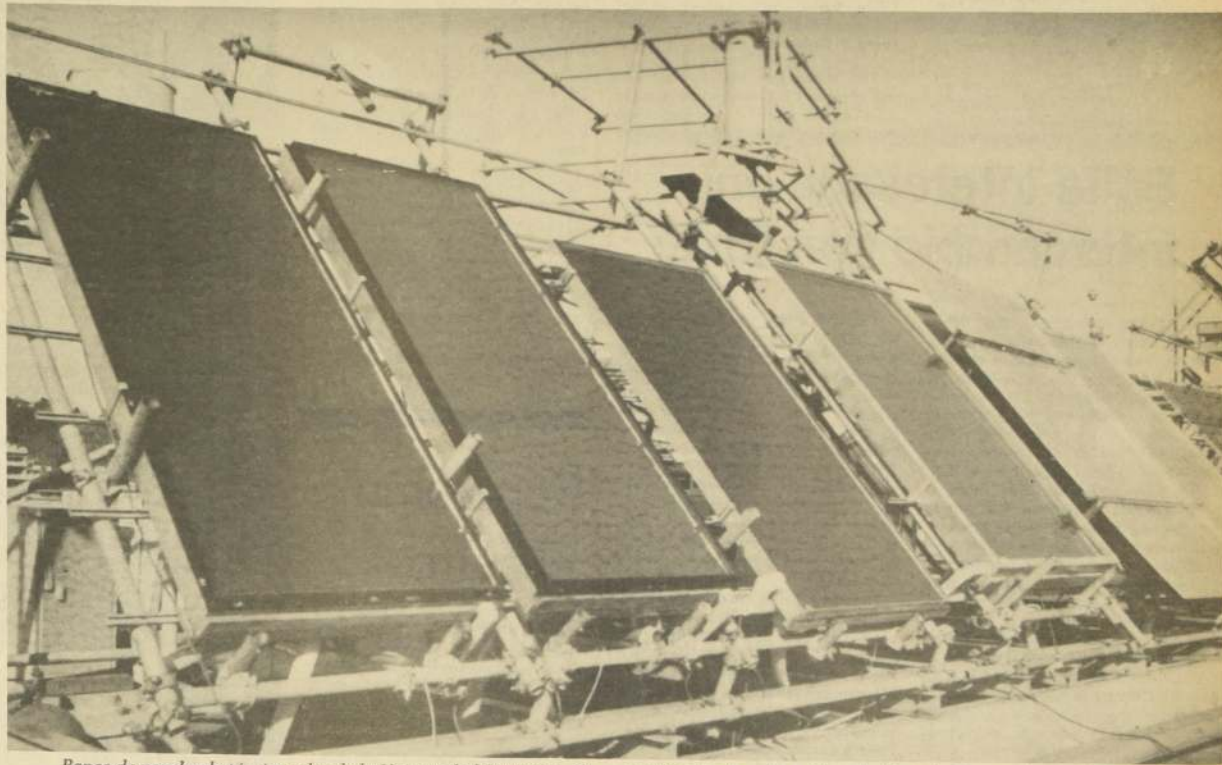
Banco de prueba de técnica solar de la Universidad Stuttgart, República Federal de Alemania, con (izquierda) colectores para la
