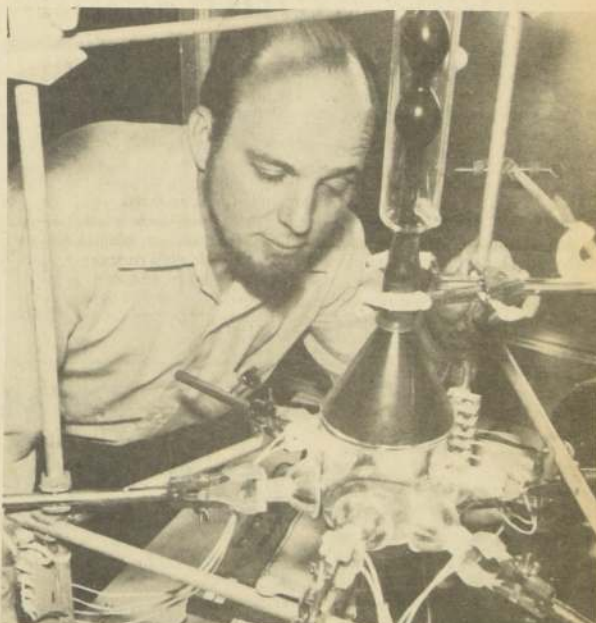
El físico del Laboratorio Berkley, California, Arlon Hunt, revisa un modelo a escala del mecanismo para el intercambio de minúsculas partículas de calor, una nueva técnica para la conservación de la energía solar. Esta técnica consiste en la irradiación de luz a una cámara que contiene pequeñas partículas de carbón que absorben la luz solar y se evaporan emitiendo calor a la atmósfera que la rodea.
