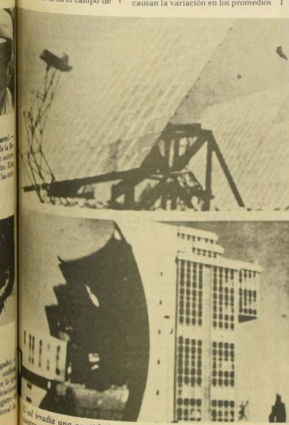
El sol irradia una cantidad de energía 26 mil veces mayor que nuestro actual requerimiento energético. Teóricamente, una mínima parte de ésta bastaría para solucionar las necesidades en la Tierra.
