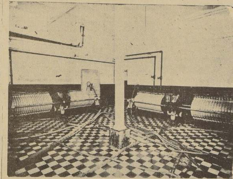
Sala de filtros para cerveza.—Fábrica Ebner
