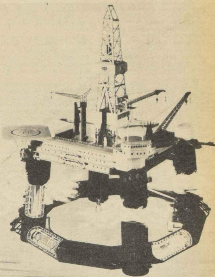
Del mar saldrá la gran mayoría de los recursos básicos para la vida del hombre en las próximas generaciones. Esta es una plataforma de prospecciones marinas especialmente diseñada para trabajar en mares embravecidos. Construida en Alemania Federal, puede operar hasta mil metros de profundidad y tiene una altura de 100 metros y un diámetro de 90.
