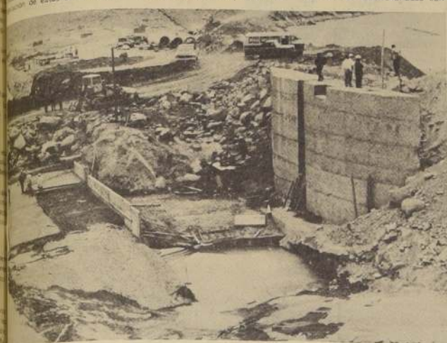
La construcción de la Toma Independiente del río Maipo, en el grabado, ha tropezado con una serie de inconvenientes derivados de las crecidas del río, en épocas climáticas desfavorables.
