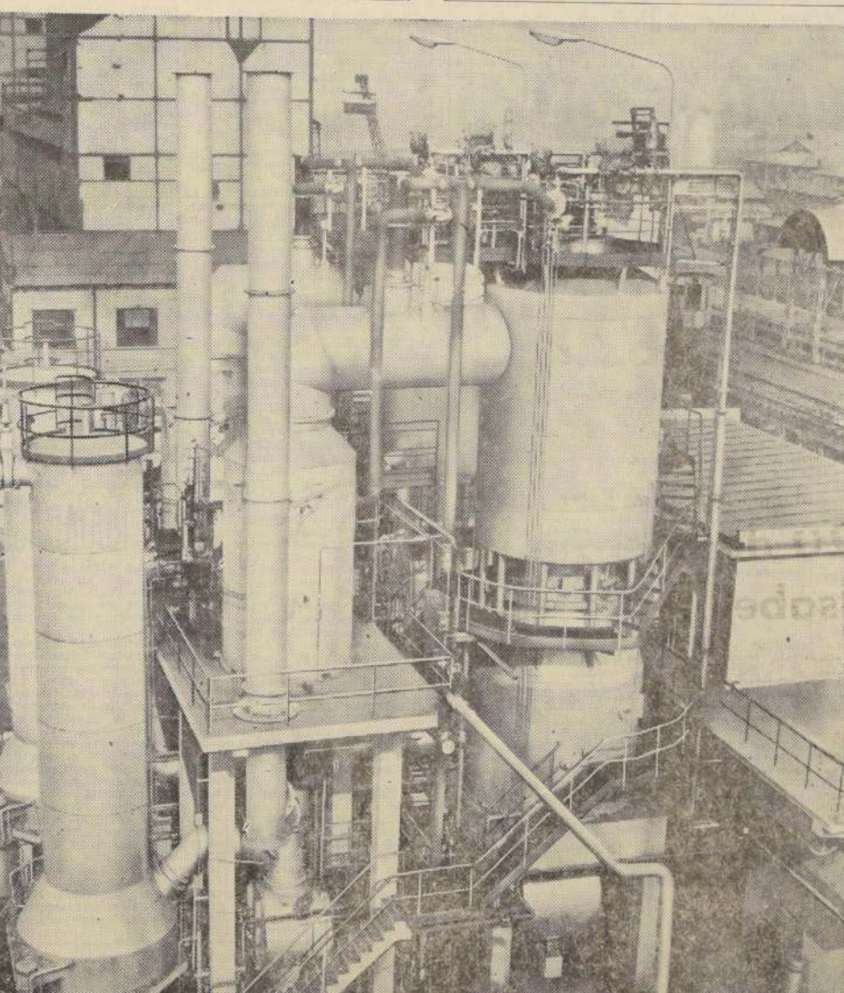
(Vista parcial de la planta de Cracking Catalítico instalada en la Fabrica San Borja).
