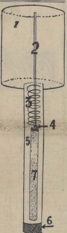
1) El cuerpo superior de la bomba infernal, compuesto de un cilindro de siete centímetros de diámetro por igual de altura.
