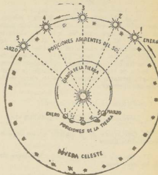
Fig. 1—Explicación del movimiento aparente del Sol sobre la bóveda celeste a lo largo del año, que da lugar a las estaciones.
