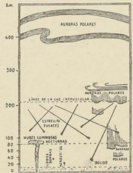
Fig. 40—Sección vertical de la atmósfera terrestre
