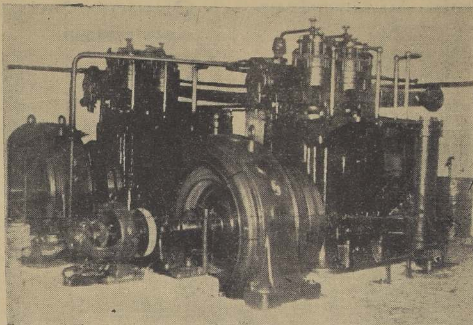
Instalación de dos Motores DIESEL "WORTHINGTON", de 120 H. P. cada uno EN LA OFICINA SALINERA "PAN DE AZÚCAR"
