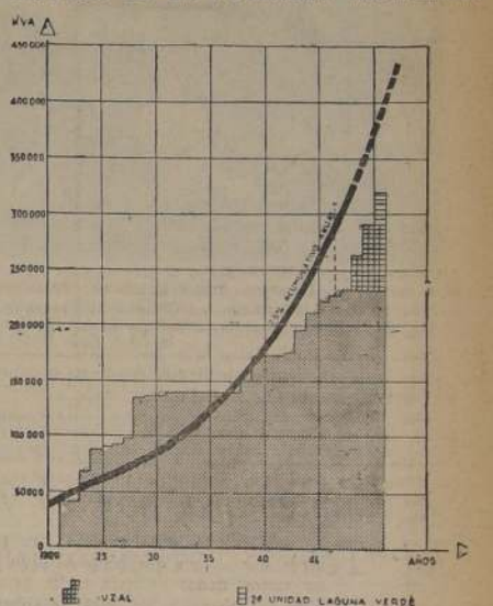
Potencia instalada en servicios públicos y particulares en las provincias de Santiago, Valparaíso y Aconcagua, y curva de previsión de la potencia necesaria
