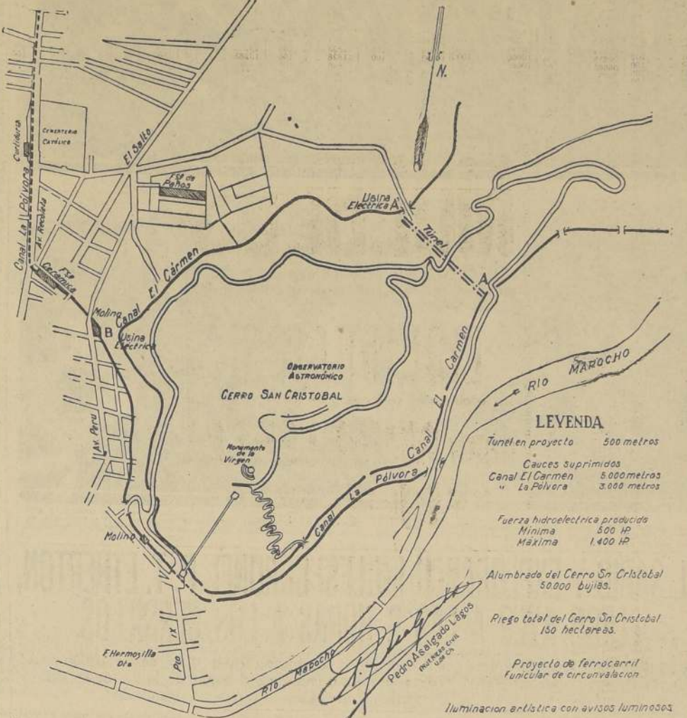
Gráfico de la obra en proyecto. La doble línea A-A' indica el recorrido del túnel
