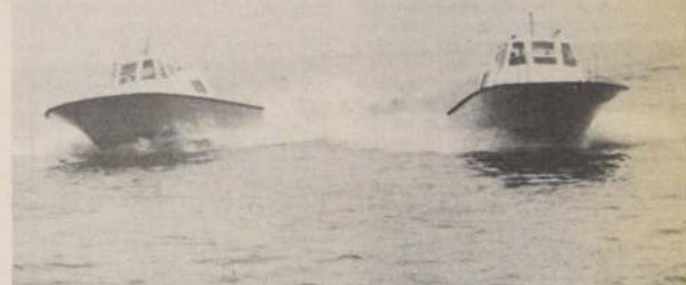
Dos lanchas de Policía Marítima, iguales a las de la foto, serán incorporadas a la Armada Nacional en los próximos días. Están hechas de resina de poliéster, reforzadas con fibra de vidrio, pudiendo desarrollar una velocidad de 17 nudos, con una autonomía de 10 horas.
