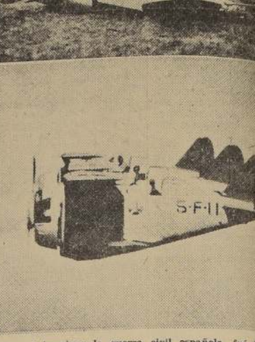
Arriba: al terminar la guerra civil española, fue llevada Francia este monoplano de caza; resultó ser uno de los "ratas" rusos que usaban los republicanos. Se trata de una máquina sumamente veloz, de forma de bala y con ametralladoras.
